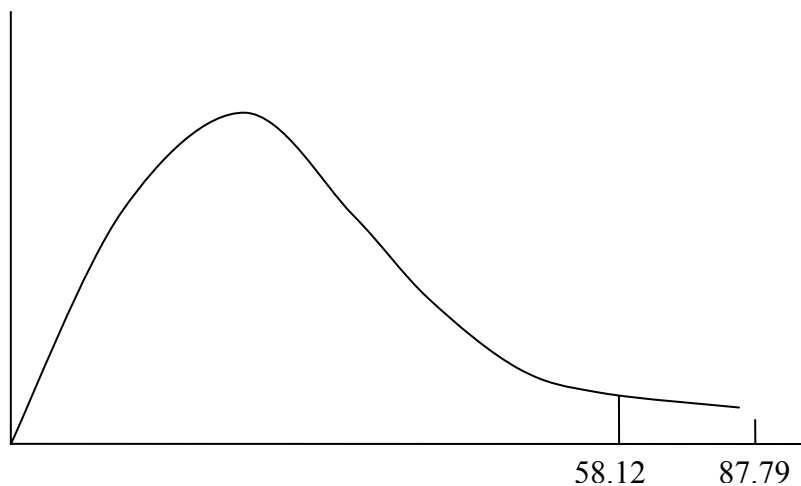
Gambar 5.3 Grafik Chi Square Pengujian III
