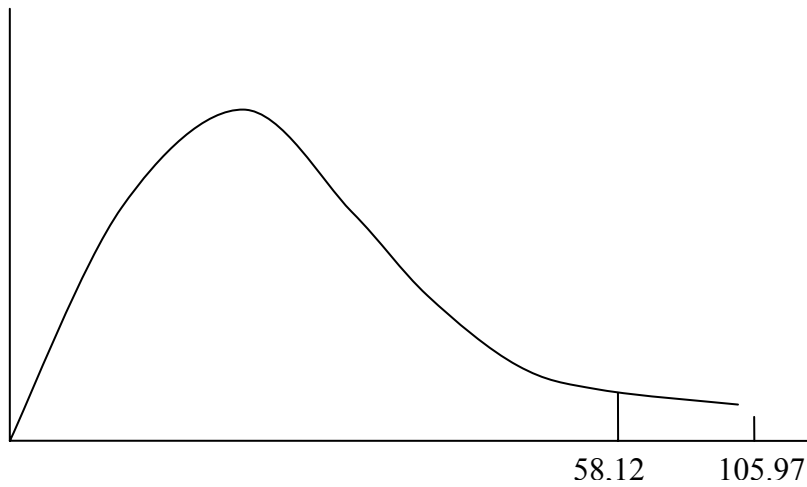
Gambar 5.2 Grafik Chi Square Pengujian II
