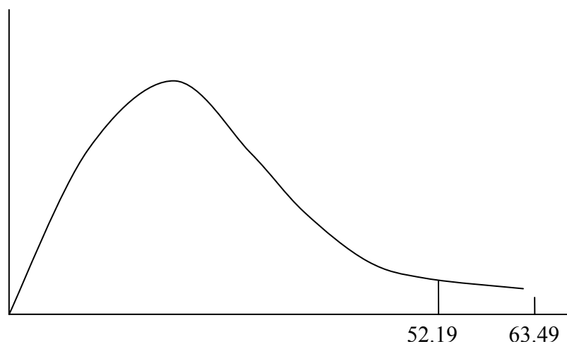
Gambar 5.5 Grafik Chi Square Pengujian V
