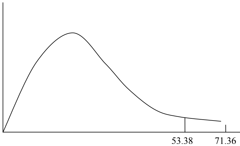
Gambar 5.4 Grafik Chi Square Pengujian IV
