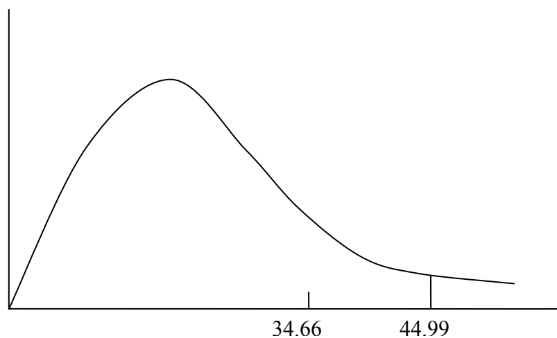
Gambar 5.8 Grafik Chi Square Pengujian VIII
