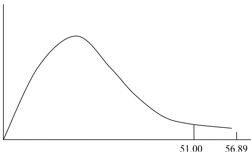
Gambar 5.6 Grafik Chi Square Pengujian VI
