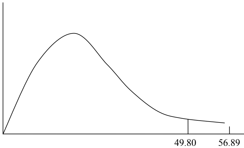
Gambar 5.7 Grafik Chi Square Pengujian VII
