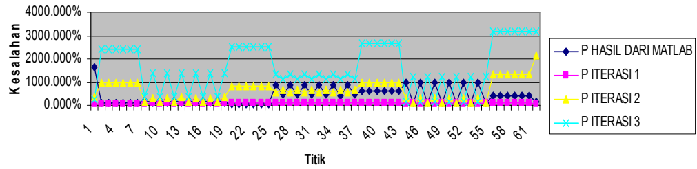
Perbandingan Kesalahan Tekanan (Magnituda) Pada Bola 62 Titik Dengan k=10 Dan r=1.08835
