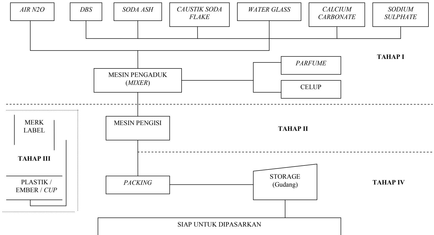
Lampiran 2: Proses Produksi Sabun Palem Cream Detergent
