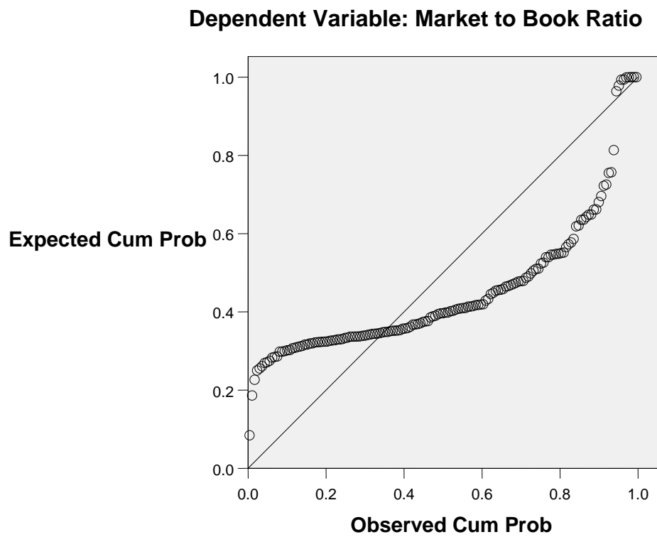
Gambar 2. Uji Normalitas
