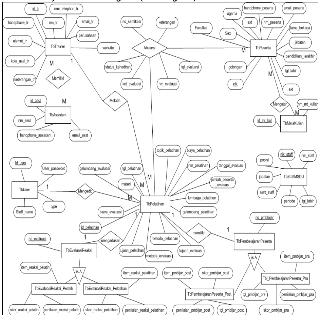
Gambar 4. ERD
