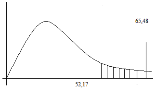
Daerah Penolakan Uji Cochran 10
