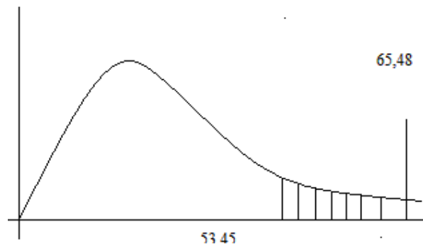
Daerah Penolakan Uji Cochran 9
