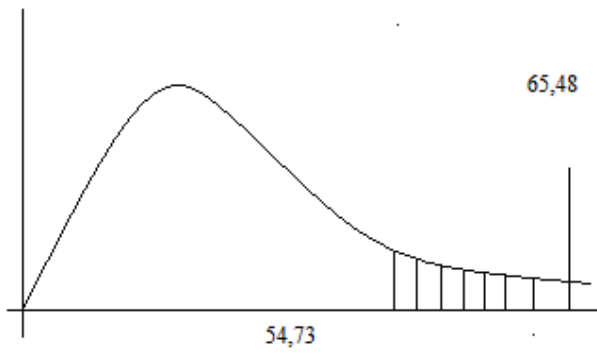
Daerah Penolakan Uji Cochran 8
