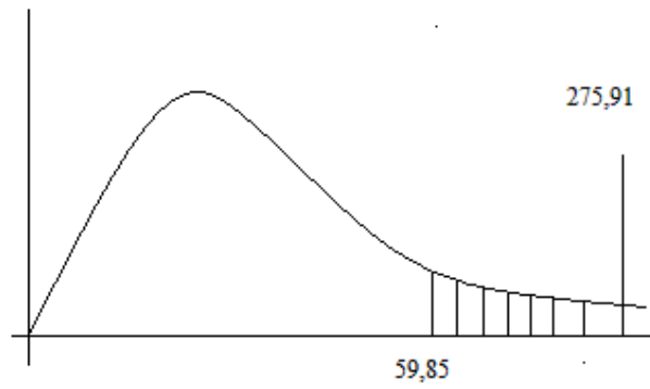
Daerah Penolakan Uji Cochran 4
