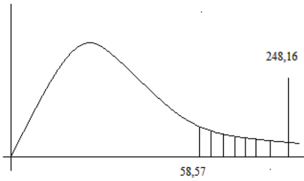
Daerah Penolakan Uji Cochran 5
