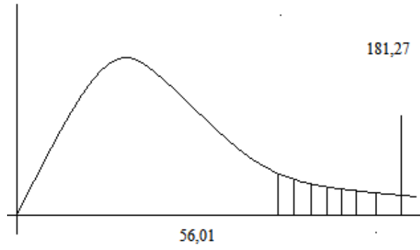
Daerah Penolakan Uji Cochran 7
