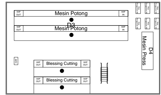
LANTAI 2
