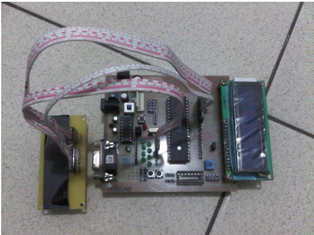
Sensor Warna TCS230 dan Pengendali Mikro ATmega16
