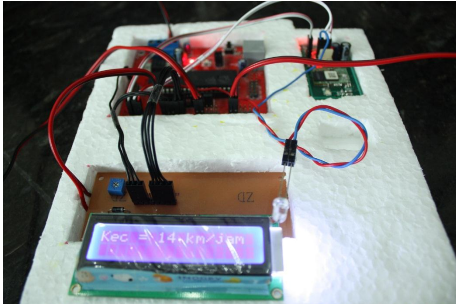
Tampilan Alat
