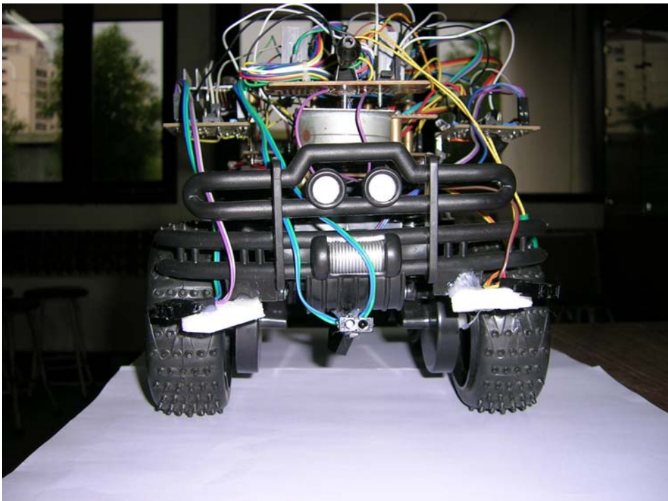
Gambar A.2 Foto Robot dilihat dari depan
