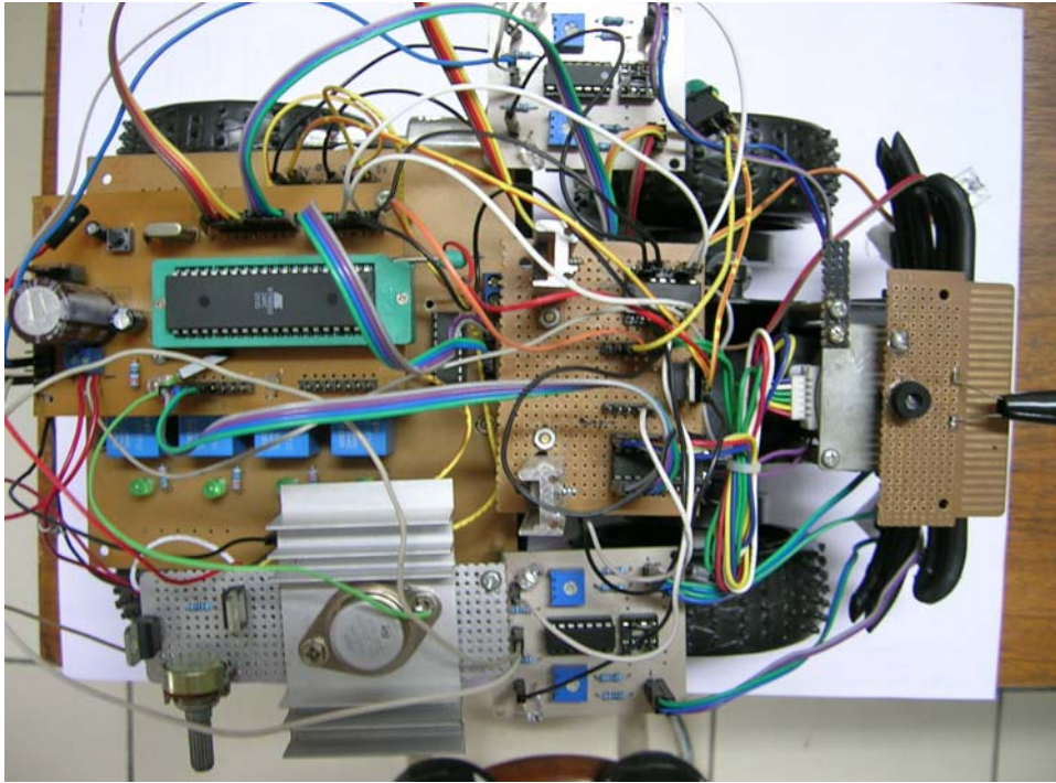
Gambar A.1 Foto Robot dilihat dari atas
