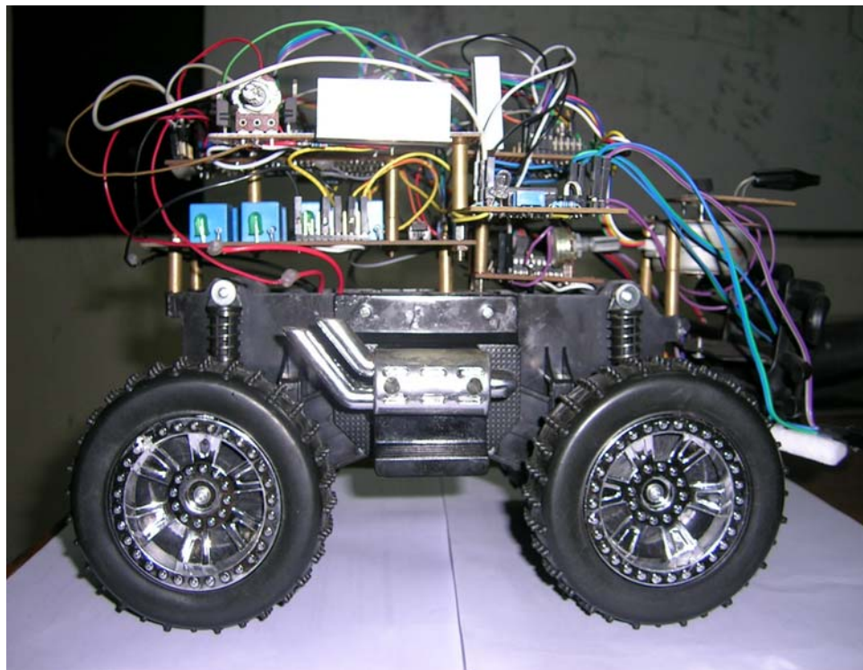
Gambar A.4 Foto Robot dilihat dari samping
