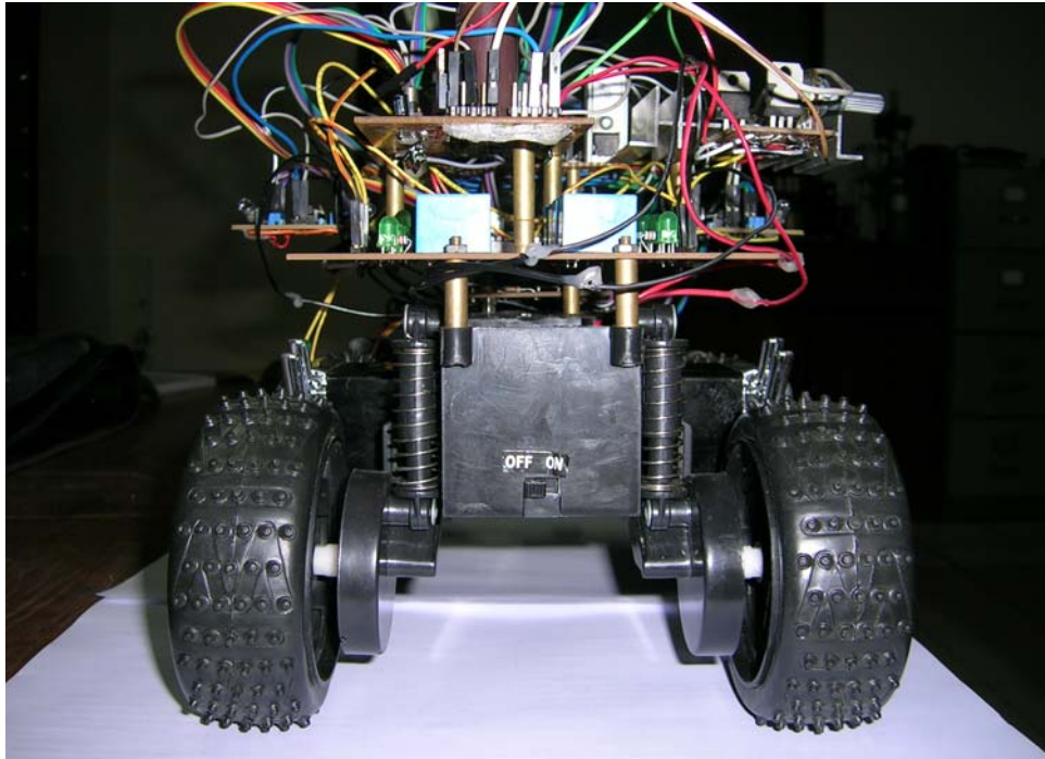
Gambar A.3 Foto Robot dilihat dari belakang
