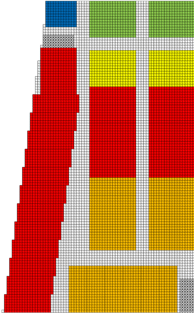
Gambar 12 Tata Letak Usulan Akhir
