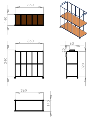
Gambar 5 Dimensi Alat Penyimpanan Kain Usulan
