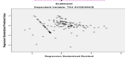
Gambar 1. Uji Heteroskedastisitas
