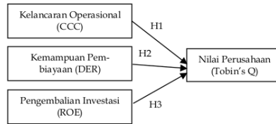
Gambar 1. Rerangka Konseptual
