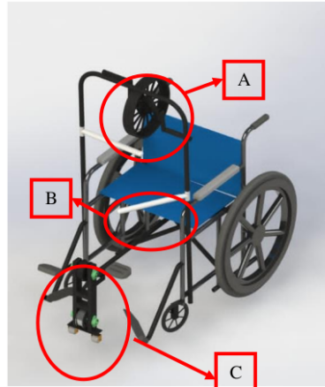
Gambar 4. Gambar 3D kursi roda terapi
