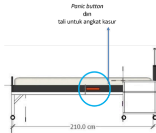
Gambar 5. Rekomendasi desain alternatif 2 fasilitas tempat tidur lansia
