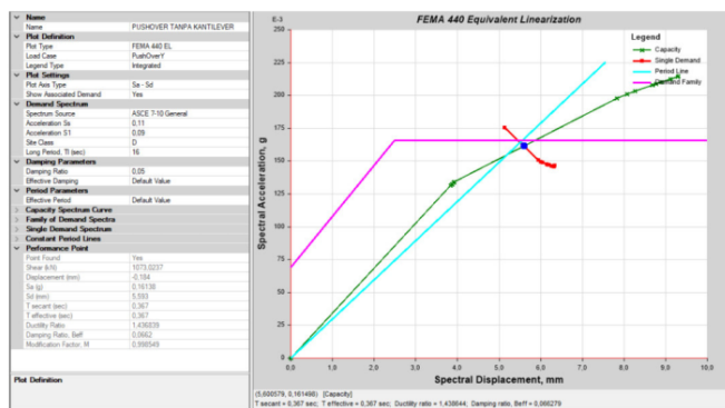
Gambar 14. Analisis kurva pushover arah Y berdasarkan FEMA 440 untuk pemodelan struktur tanpa kantilever
