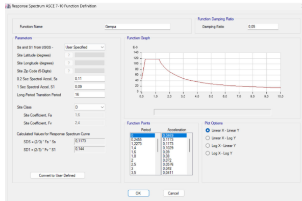
Gambar 7. Kurva spektrum respon rencana
