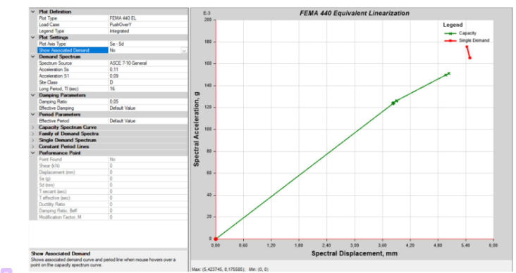
Gambar 12. Analisis kurva pushover arah Y berdasarkan FEMA 440 untuk pemodelan struktur dengan kantilever
