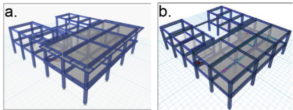
Gambar 6. (a) Denah 3D struktur dengan kantilever; (b) Denah 3D struktur utama tanpa kantilever
