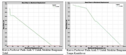
Gambar 10. Perbandingan kurva pushover arah Y
