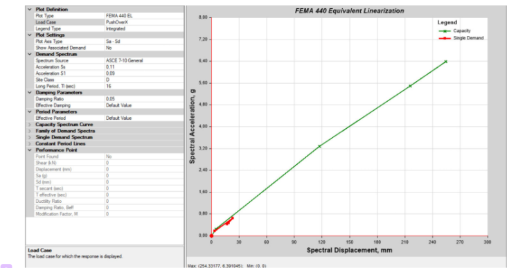
Gambar 11. Analisis kurva pushover arah X berdasarkan FEMA 440 untuk pemodelan struktur dengan kantilever
