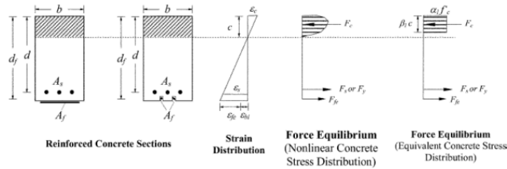
Gambar 2.2 Hubungan Diagram Tegangan Regangan Perkuatan Lentur
