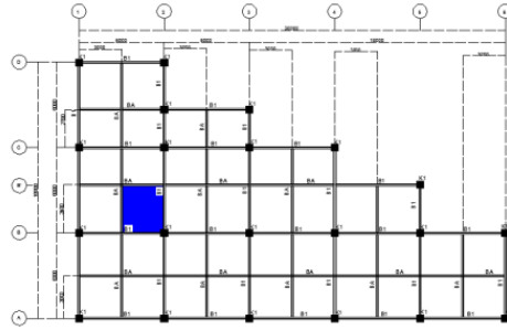
Gambar 3.2 Lokasi Pelat Lt.4 (1'2-BB')
