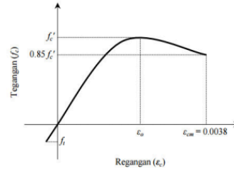
Gambar 2.1 Hubungan Tegangan Regangan Beton Menurut Hognestad
