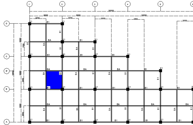
Gambar 3.2 Lokasi Pelat Lt.4 (1'2-BB')
