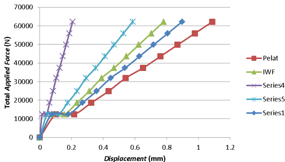
Gambar 4.1 Total Applied Load vs Displacement perbandingan antara pelat lantai, Pelat Lantai + FRP1, Pelat Lantai + FRP2, Pelat Lantai + FRP3, Pelat Lantai + IWF
