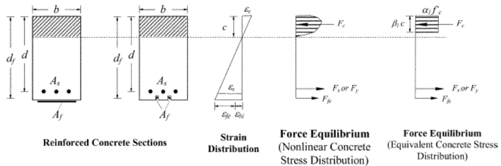
Gambar 2.2 Hubungan Diagram Tegangan Regangan Perkuatan Lentur
