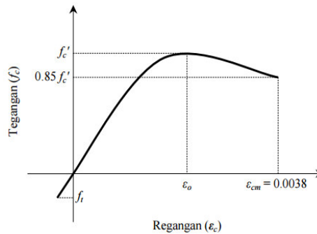
Gambar 2.1 Hubungan Tegangan Regangan Beton Menurut Hognestad
