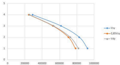
Gambar 4.2 Persyaratan 0,85 V_{sy} \leq V_{dy} (Arah Y)
