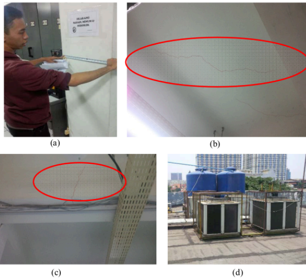
Gambar 3.1 (a) Pengukuran dimensi struktur kolom, (b) Retak pelat lantai 4, (c) Retak balok induk lantai 4, (d) Beban pada dak atap
