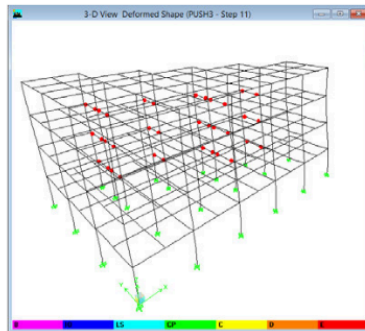
Gambar 4.6 Tingkat Kerusakan Struktur Gedung X pada PUSH 3 Step 11
