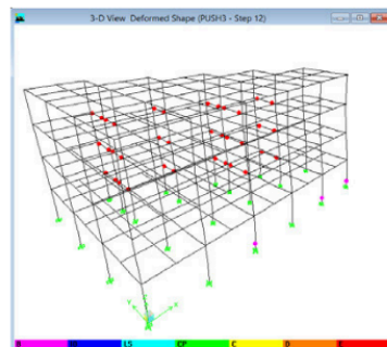
Gambar 4.7 Tingkat Kerusakan Struktur Gedung X pada PUSH 3 Step 12 .
