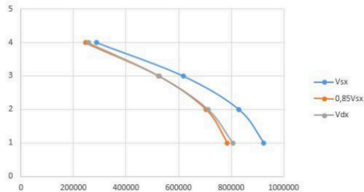
Gambar 4.1 Persyaratan 0,85 V_{sx} \leq V_{dx} (Arah X)
