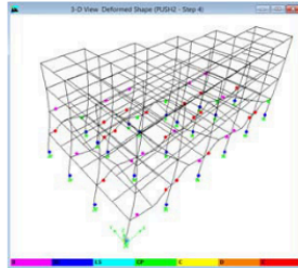
Gambar 4.3 Tingkat Kerusakan Struktur Gedung X pada PUSH 2 Step 4
