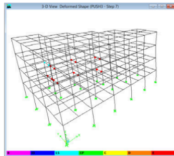
Gambar 4.5 Tingkat Kerusakan Struktur Gedung X pada PUSH 3 Step 7
