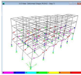
Gambar 4.4 Tingkat Kerusakan Struktur Gedung X pada PUSH 2 Step 7
