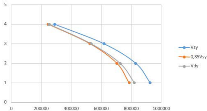
Gambar 4.2 Persyaratan 0,85 V_{s_x} \leq V_{d_x} (Arah Y)
