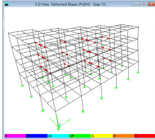
Gambar 4.6 Tingkat Kerusakan Struktur Gedung X pada PUSH 3 Step
