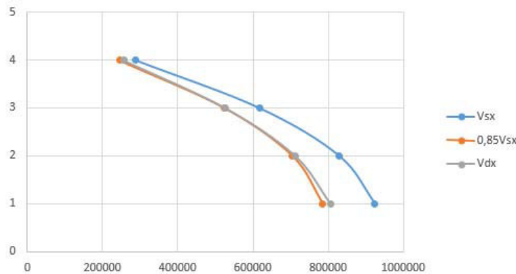
Gambar 4.1 Persyaratan 0,85 V_{s_x} \leq V_{d_x} (Arah X)
