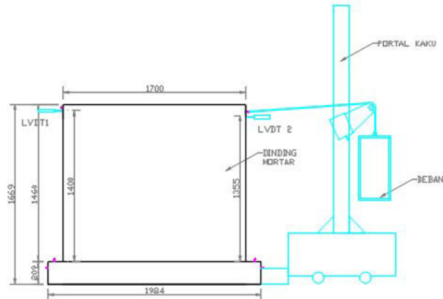
Gambar 6 Skema Pengujian Dinding Mortar Cor di Tempat
