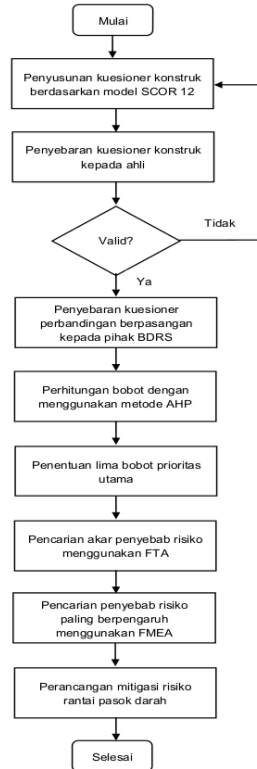
Gambar 1. Metodologi penelitian
