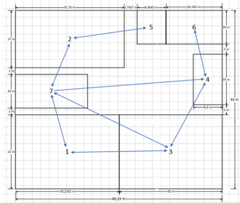
Gambar 6. Gambar tata letak usulan
