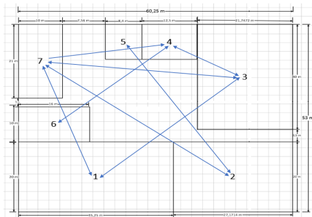
Gambar 2. Gambar tata letak awal
