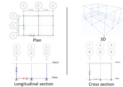
Fig. 9. ETABS design
