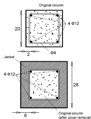
Gambar 6. Penambahan dimensi kolom
