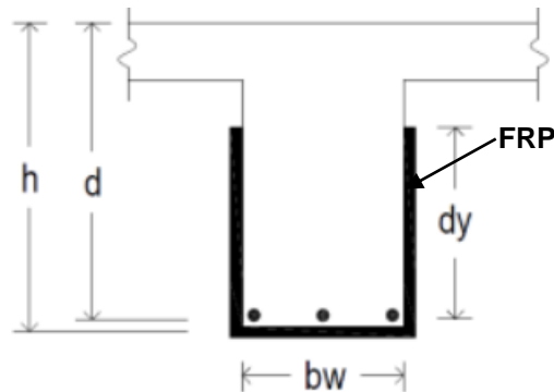
Gambar 7. Penambahan FRP untuk kegagalan geser pada balok
