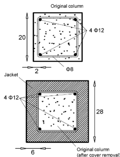
Gambar 6. Penambahan dimensi kolom
