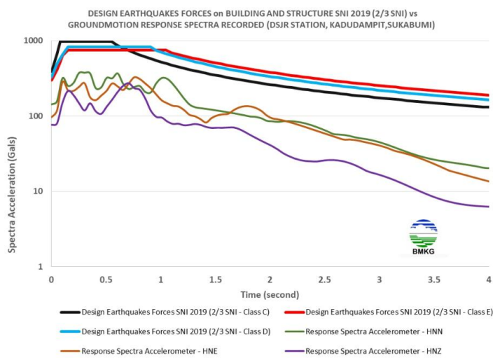
Gambar 4. Respon spektra stasiun KJCR dan respon spektra desain pada lokasi di Cianjur (Sumber BMKG)
