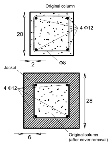
Gambar 6. Penambahan dimensi kolom
