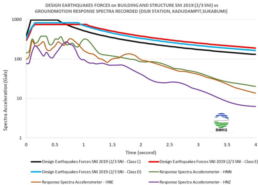
Gambar 4. Respon spektra stasiun KJCR dan respon spektra desain pada lokasi di Cianjur (Sumber: BMKG)
