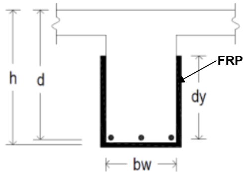
Gambar 7. Penambahan FRP untuk kegagalan geser pada balok
