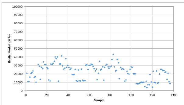
Gambar 4. Data modulus elastisitas dinamik hasil pengujian sampel rumah tinggal di kota Manado (Pranata dan Rusli, 2015).
