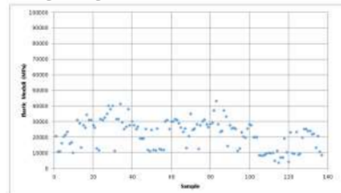
Gambar 4. Data Modulus Elastisitas Dinamik Hasil Pengujian Sampel Rumah Tinggal di Kota Manado (Pranata & Rusli, 2015).
