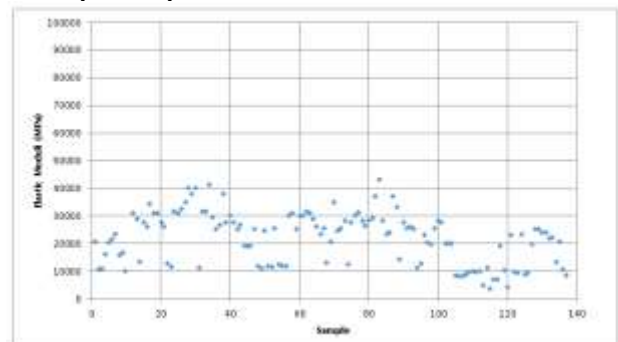
Gambar 4. Data Modulus Elastisitas Dinamik Hasil Pengujian Sampel Rumah Tinggal di Kota Manado (Pranata & Rusli, 2015).
