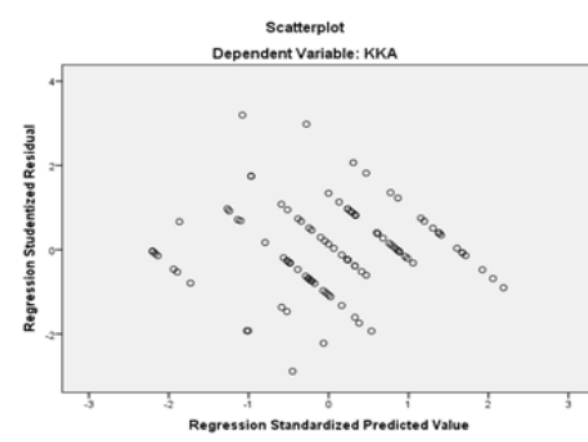
Gambar 1. Uji Heteroskedastisitas
