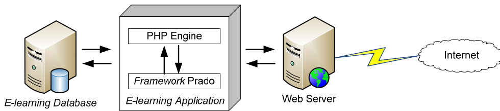
Gambar 2 Implementasi Arsitektur Aplikasi
