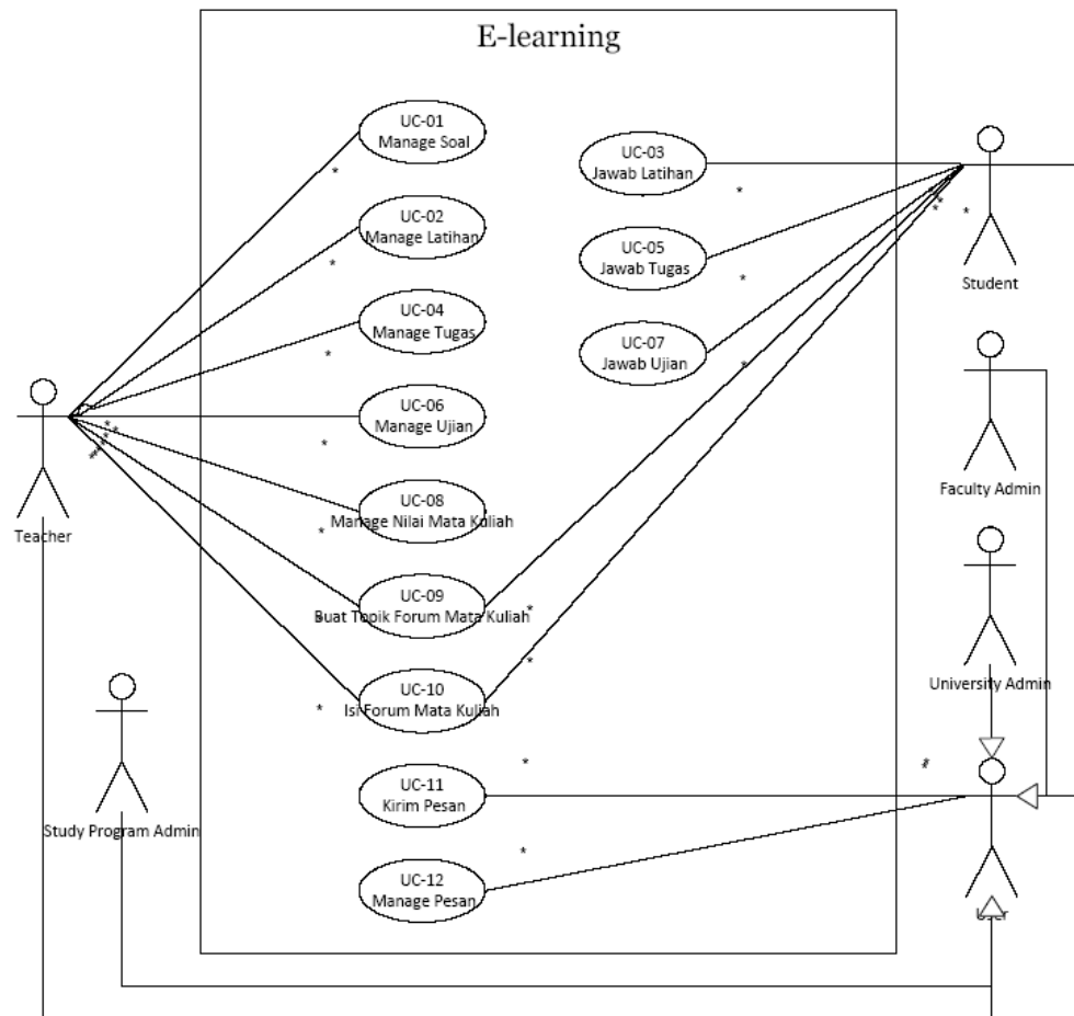
Gambar 3 Use Case Diagram Aplikasi
