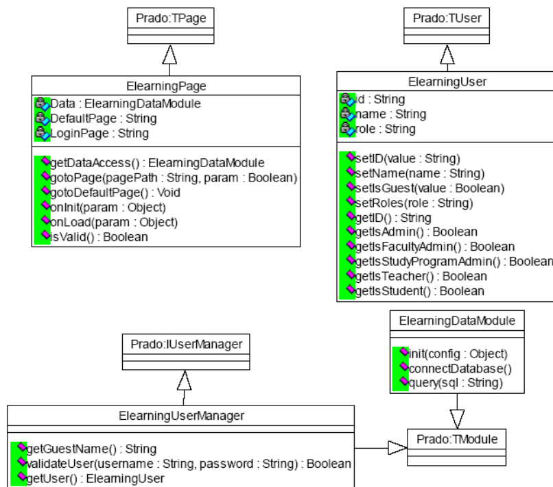
Gambar 4 Class Diagram Komponen Dasar Aplikasi
