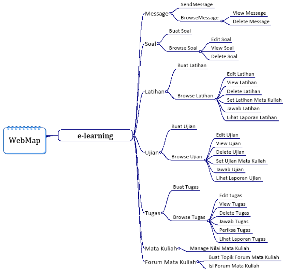
Gambar 7 Struktur Halaman Web Site Aplikasi E-learning
