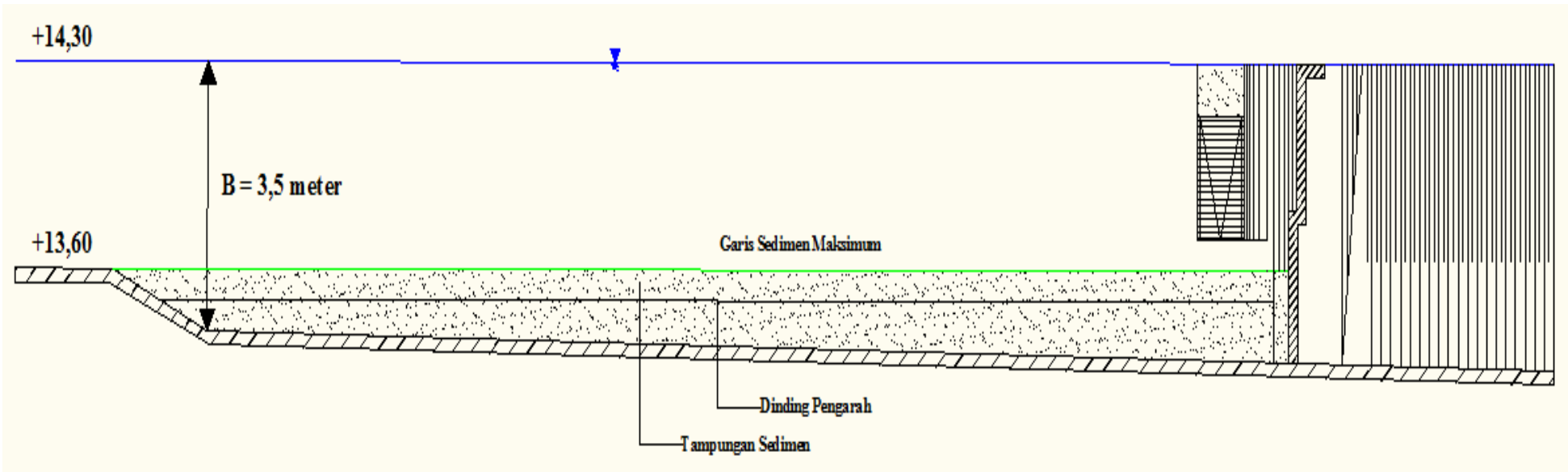
Lampiran L.2 Potongan Memanjang Bangunan Penangkap Sedimen
