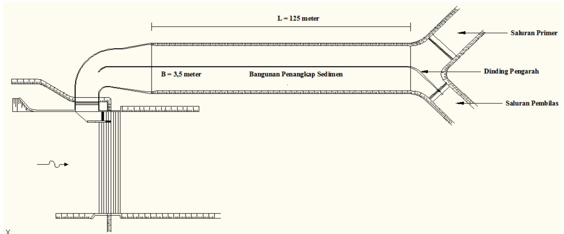
Lampiran L.1 Tampak Atas Bangunan Penangkap Sedimen
