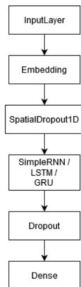
Gambar 5. Arsitektur RNN , LSTM , dan GRU
