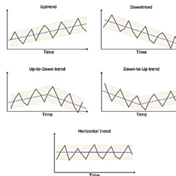
Gambar 1. Tren dalam data time series
