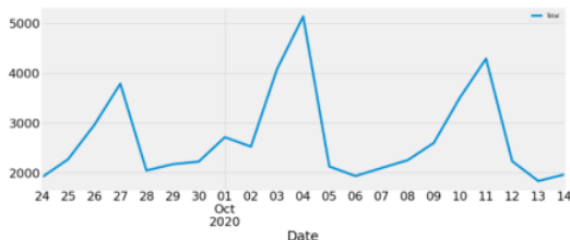
Gambar 6. Visualisasi data visitor
