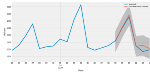
Gambar 11. Hasil validasi prediksi
