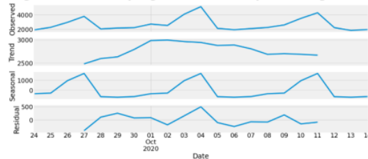
Gambar 7. Hasil dekomposisi data visitor
