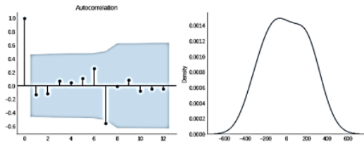
Gambar 19. Plot autokorelasi dan histogram model Holt Winter
