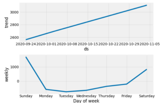
Gambar 22. Visualisasi komponen hasil prediksi
