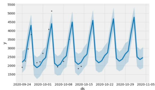
Gambar 21. Visualisasi hasil prediksi
