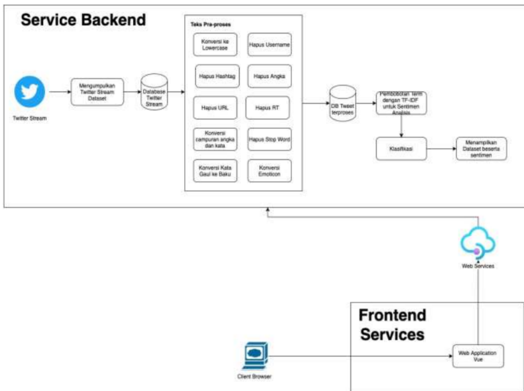
Gambar 2. Arsitektur aplikasi berbasis microservices
