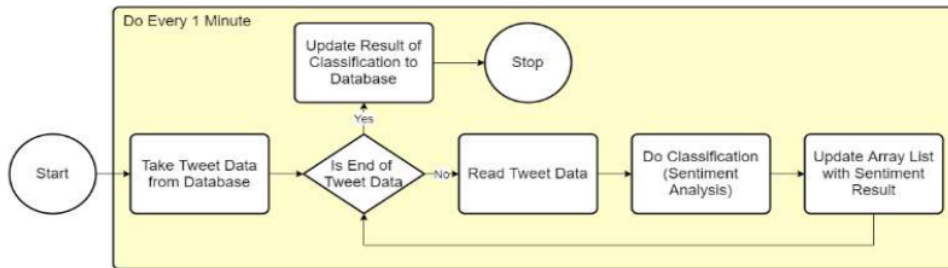
Gambar 5. Ilustrasi proses klasifikasi analisis sentimen
