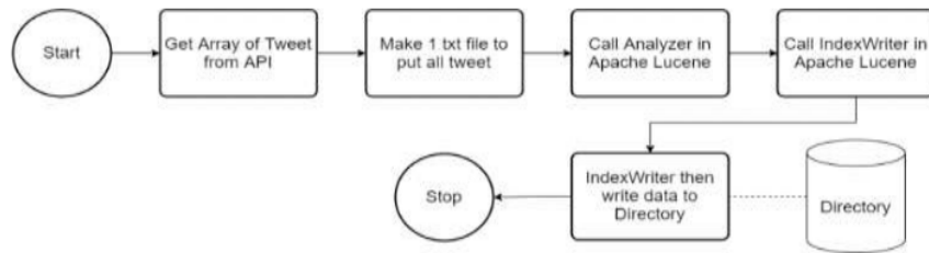
Gambar 4. Ilustrasi penggunaan Lucene untuk proses indexing
