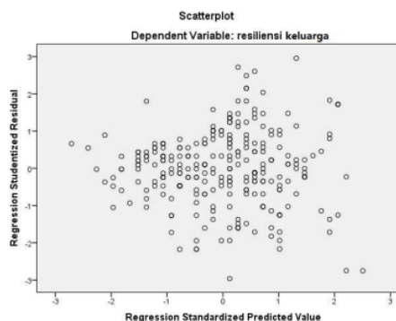
Gambar 1. Scatterplot uji heteroskedastisitas
