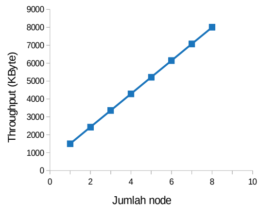
Gambar 3. Throughput sistem terhadap jumlah node
