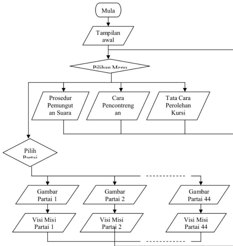
9 Gambar 3. Diagram alir
