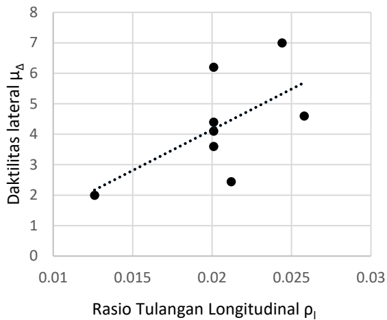
Gambar 6 Korelasi rasio tulangan longitudinal dengan daktilitas lateral
