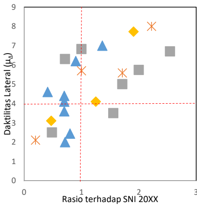
Gambar 11 Rasio Tulangan Benda Uji Terhadap Nilai Minimum SNI 20XX
