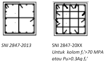
Gambar 2 Perbedaan Detailing Tulangan Pengekaung Kolom Persegi SNI 2013 dan SNI 20XX
