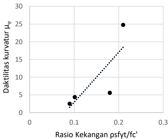
Gambar 7 Pengaruh penambahan penggunaan cross ties pada tulangan pengekan (L16-T1 sampai T3) terhadap daktilitas kurvatur
