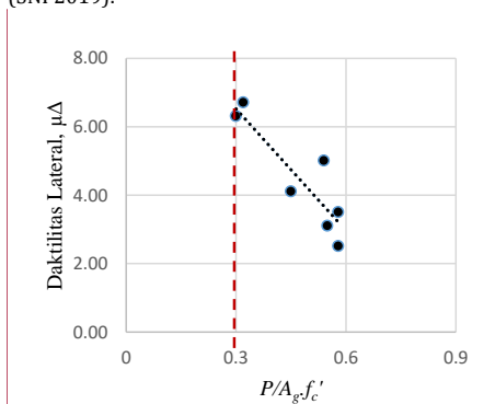
Gambar 9 Pengaruh Beban Aksial pada Daktilitas Lateral Kolom
