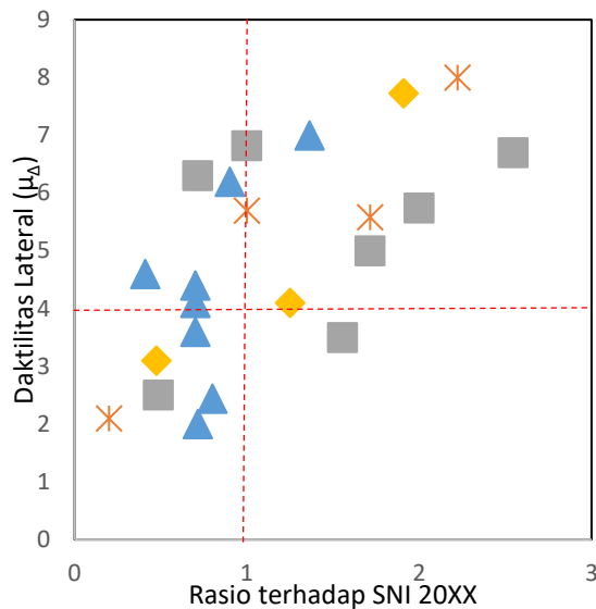
Gambar 11 Rasio Tulangan Benda Uji Terhadap Nilai Minimum SNI 20XX
