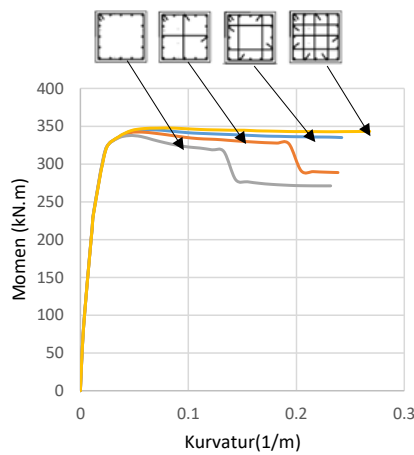
Gambar 8 Hubungan momen-kurvatur pada peningkatan jumlah tulangan pengikat
