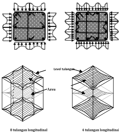
Gambar 1 Distribusi Tegangan Lateral yang Terbentuk Pada Berbagai Konfigurasi Tulangan Pengekaung
