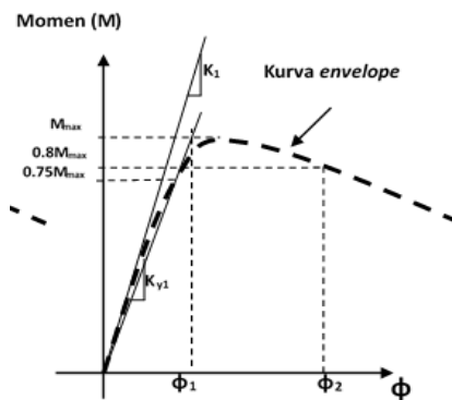
Gambar 4 Kurva definisi daktilitas
