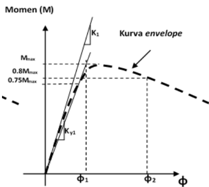
Gambar 4 Kurva definisi daktilitas Sumber: Brachmann et al - 2004
