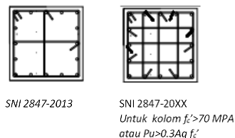
Gambar 2 Perbedaan Detailing Tulangan Pengekang Kolom Persegi SNI 2013 dan SNI 20XX
