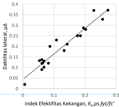
Gambar 5 Korelasi Indeks Efektif Kekangan terhadap kemampuan daktilitas lateral kolom
