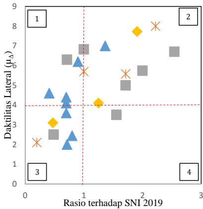
Gambar 11 Rasio Tulangan Benda Uji Terhadap Nilai Minimum SNI 2847-2010
