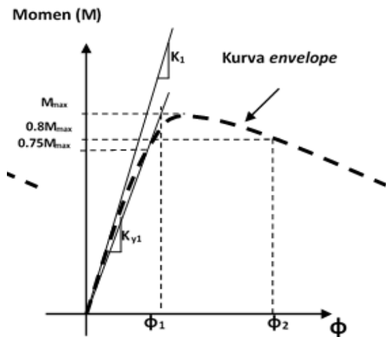
Gambar 4 Kurva definisi daktilitas
