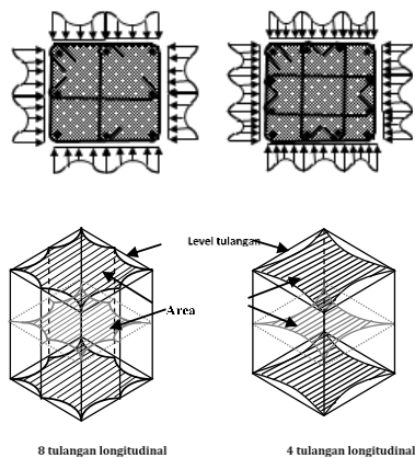
Gambar 1 Distribusi Tegangan Lateral yang Terbentuk Pada Berbagai Konfigurasi Tulangan Pengekang
