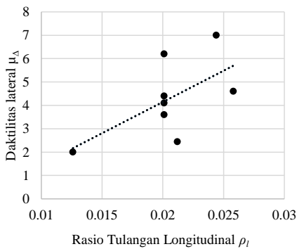
Gambar 6 Korelasi rasio tulangan longitudinal dengan daktilitas lateral
