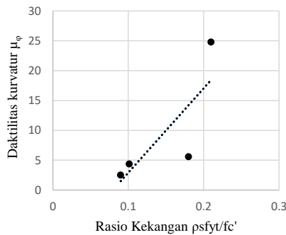
Gambar 7 Pengaruh penambahan penggunaan crossties pada tulangan pengeang (L16-T1 sampai T3) terhadap daktilitas kurvatur
