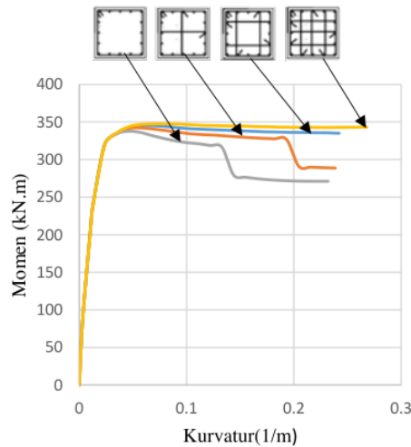
Gambar 8 Hubungan Momen-Kurvatur pada Peningkatan Jumlah Tulangan Pengikat
