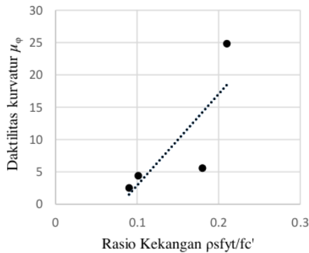
Gambar 7 Pengaruh Penambahan Penggunaan Crosssties pada Tulangan Pengekang (L16-T1 Sampai T3) terhadap Daktilitas Kurvatur
