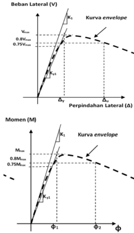
Gambar 4 Kurva Definisi Daktilitas Sumber: (Brachmann et al. 2004)
