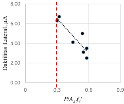
Gambar 9 Pengaruh Beban Aksial pada Daktilitas Lateral Kolom
