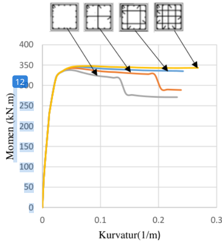
Gambar 8 Hubungan Momen-Kurvatur pada Peningkatan Jumlah Tulangan Pengekat
