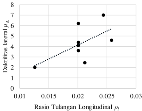
Gambar 6 Korelasi Rasio Tulangan Longitudinal dengan Daktilitas Lateral
