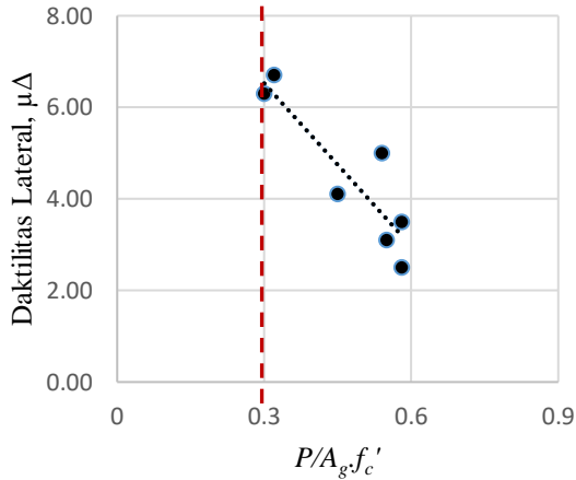
Gambar 9 Pengaruh Beban Aksial pada Daktilitas Lateral Kolom
