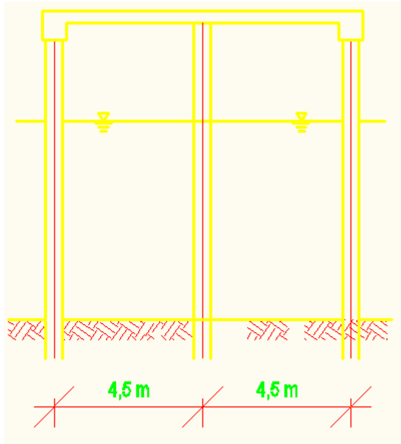
Gambar L.1 Denah Tampak Depan Struktur Dermaga
