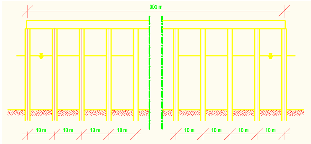
Gambar L.2 Denah Tampak Samping Struktur Dermaga
