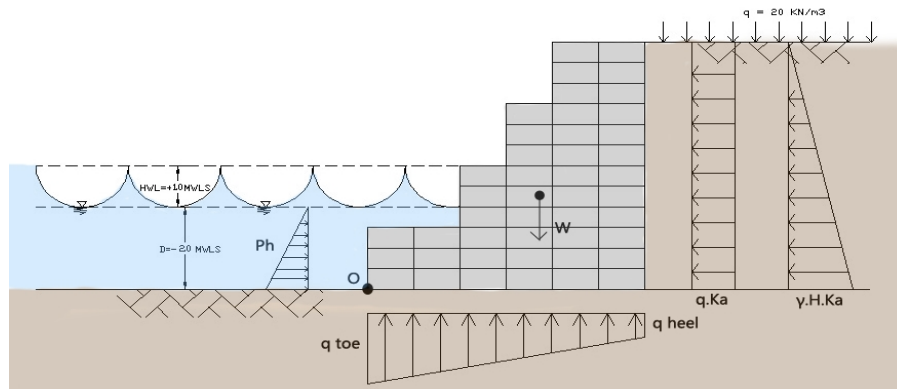
Gambar 4. Momen O sebagai momen guling
