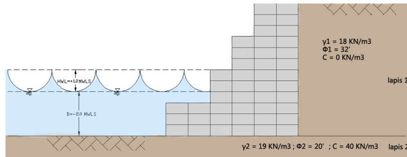
Gambar 1. Struktur Pelindung Pantai
