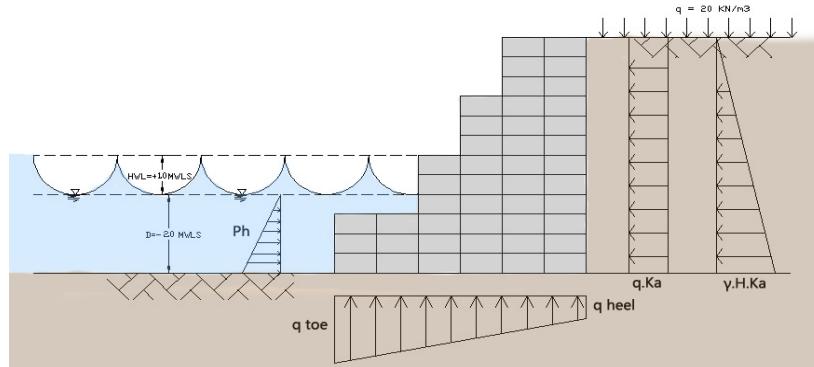
Gambar 3. Gaya – gaya yang bekerja
