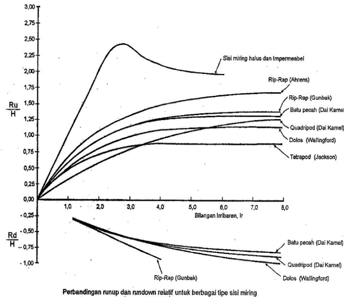
Gambar 2. Gelombanag runup untuk berbagai tipe sisi miring
