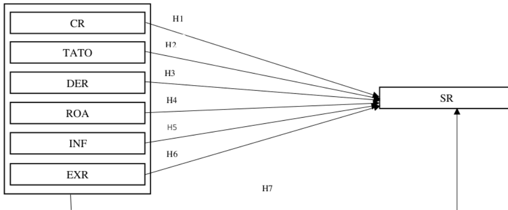
Gambar 2. Kerangka Konseptual
