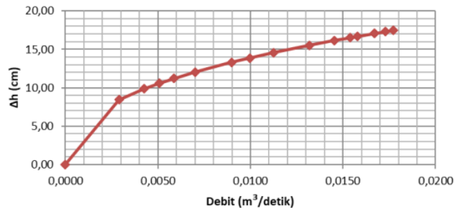
Gambar 2 Lengkung Debit
