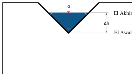
Gambar 1 Tampak Depan Alat Ukur Thomson
