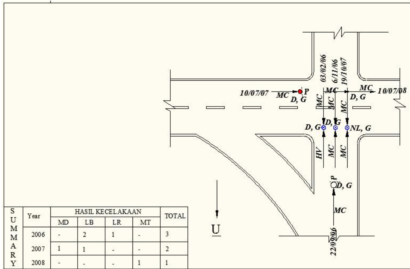
L.8 Diagram Tabrakan simpang 4 lengan jl. Moh Toha – jl. Soekarno Hatta
