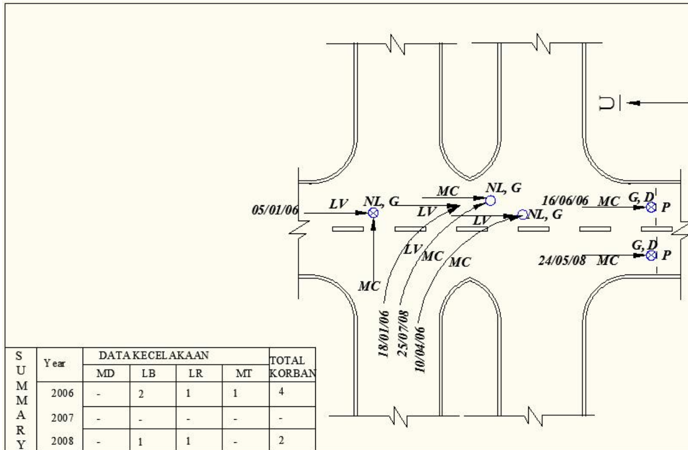
L.1 Diagram tabrakan simpang 4 lengan jl. Pasteur – jl. Cihampelas
