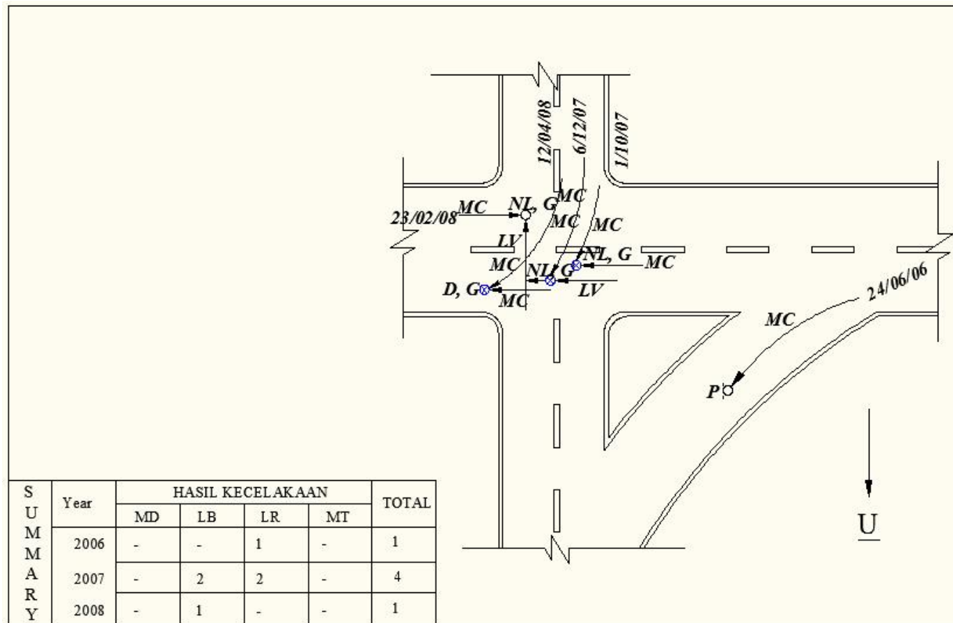
L.5 Diagram Tabrakan simpang 4 lengan jl. Gatot Subroto – jl. Lingkar Selatan
