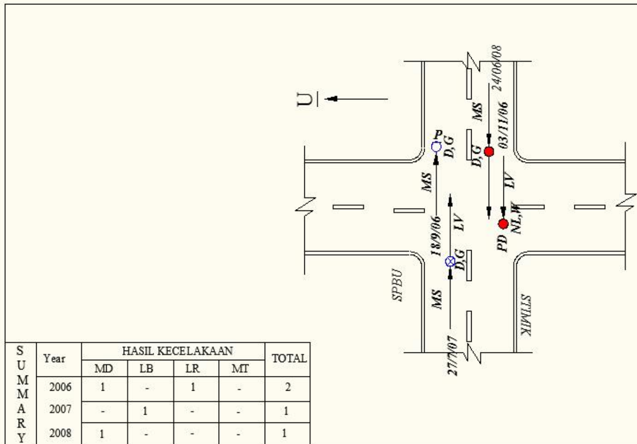
L.10 Diagram Tabrakan simpang 4 lengan jl. Soekarno Hatta (depan STIMIK)
