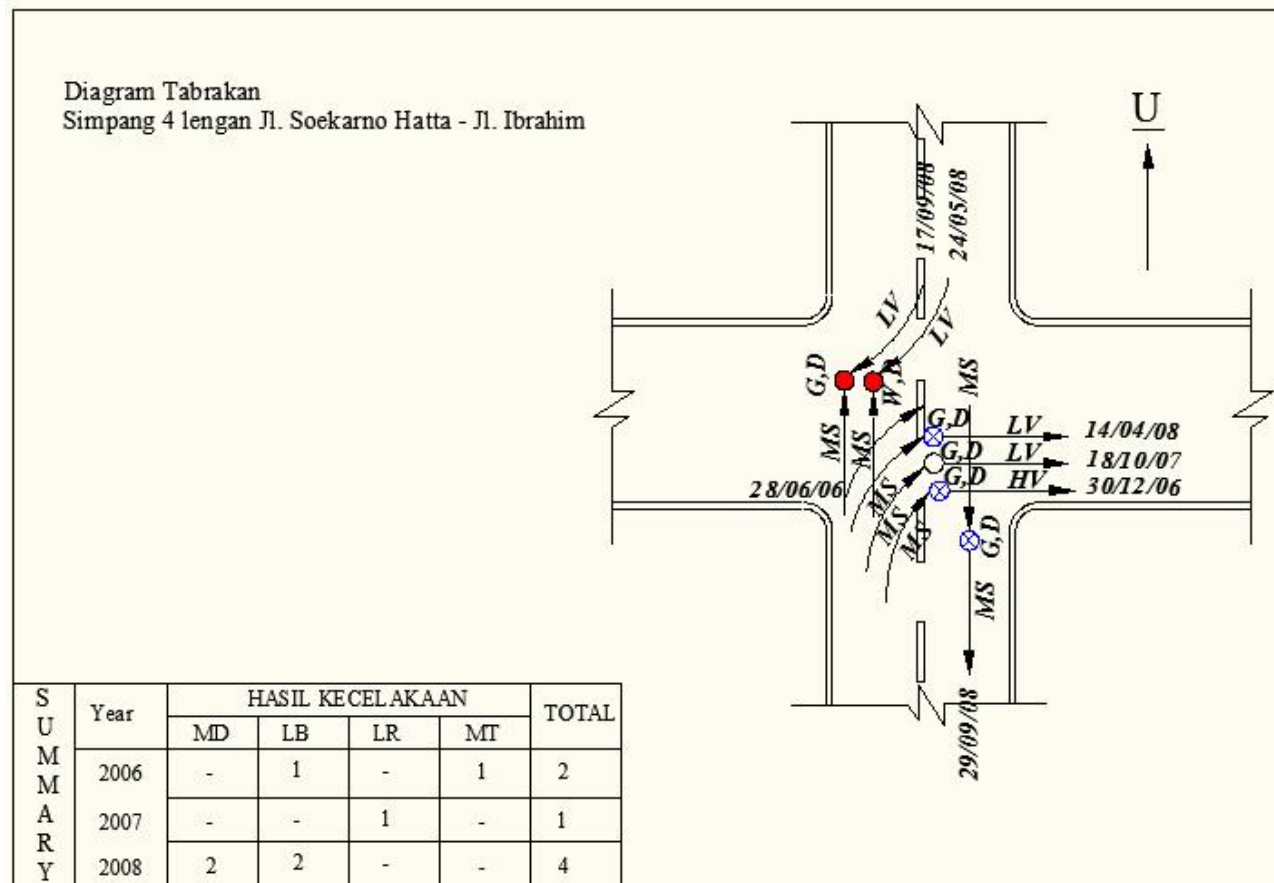
L.11 Diagram Tabrakan simpang 4 lengan jl. Soekarno Hatta – jl. Ibrahim
