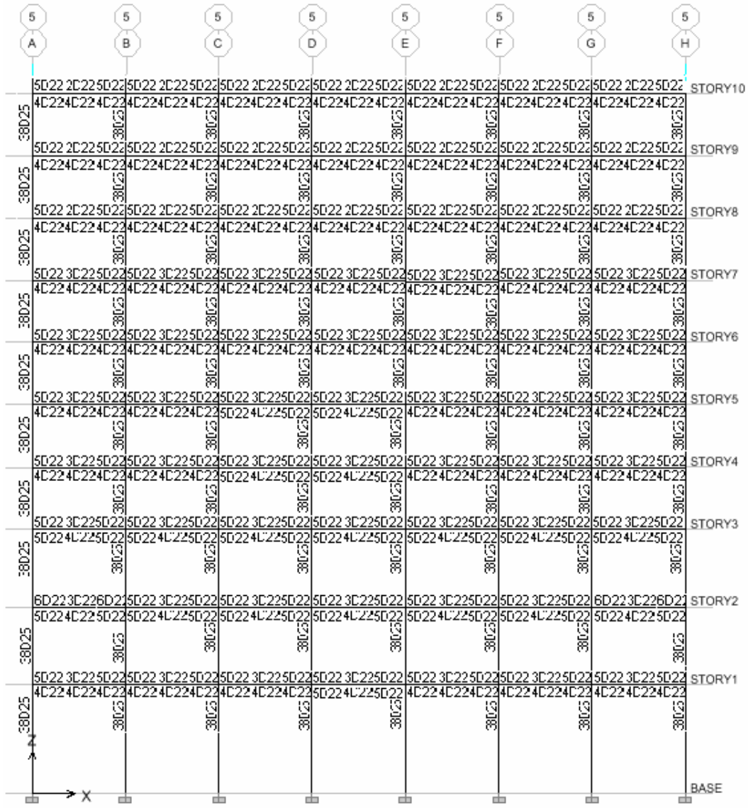
Tulangan Perlu Portal 5 (A-H)
