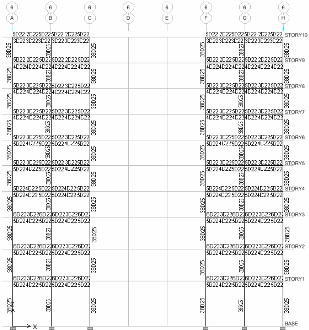
Tulangan Perlu Portal 6 (A-H)
