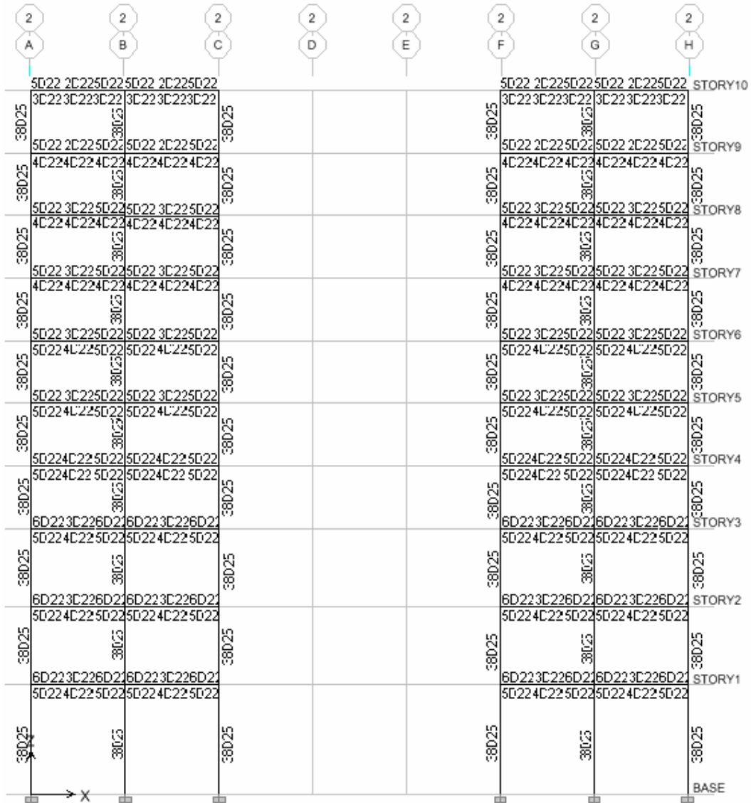
Tulangan Perlu Portal 2 (A-H)
