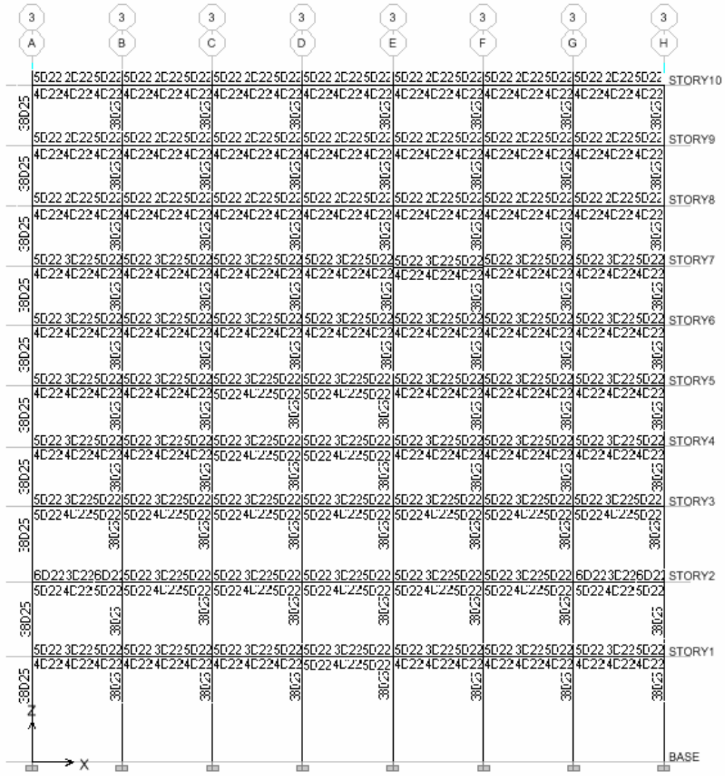
Tulangan Perlu Portal 3(A-H)
