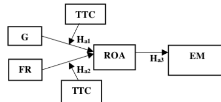
Gambar 1. Kerangka Penelitian
